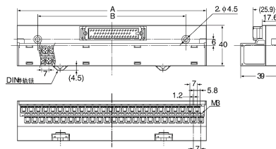
尺寸表
