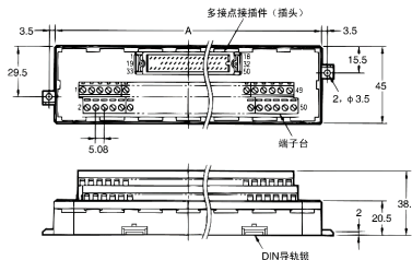
外形尺寸
