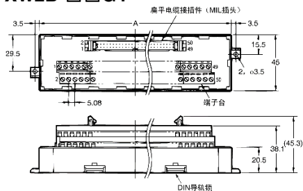
尺寸表
