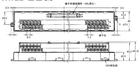
尺寸表
