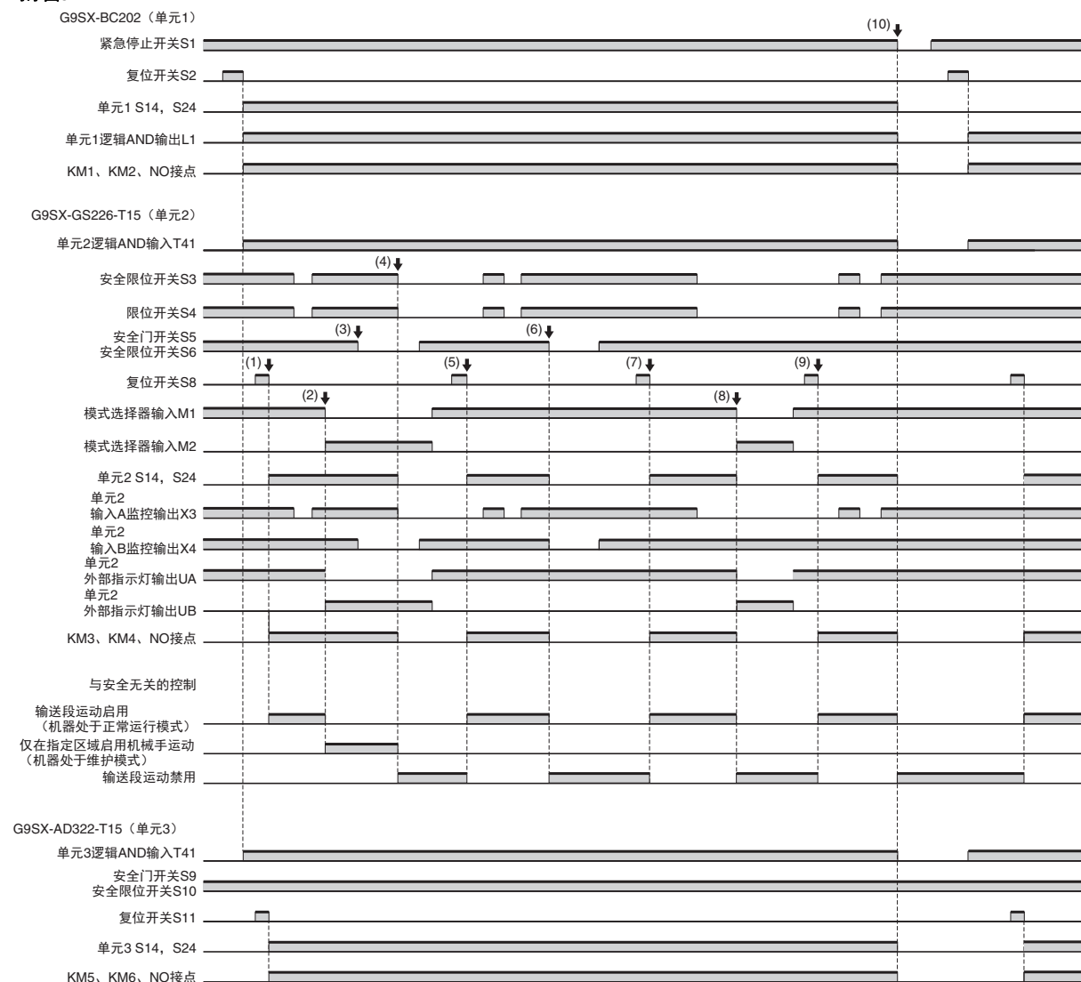
时序图3
