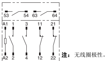
G7Z-2A2B-20Z
