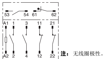
G7Z-2A2B-11Z
