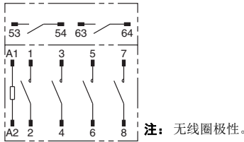
G7Z-3A1B-20Z-R
