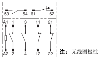
G7Z-2A2B-11Z-R
