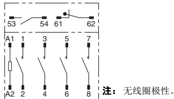
G7Z-3A1B-11Z
