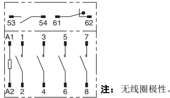
G7Z-3A1B-11Z-R
