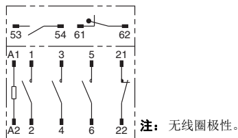
G7Z-2A2B-11Z
