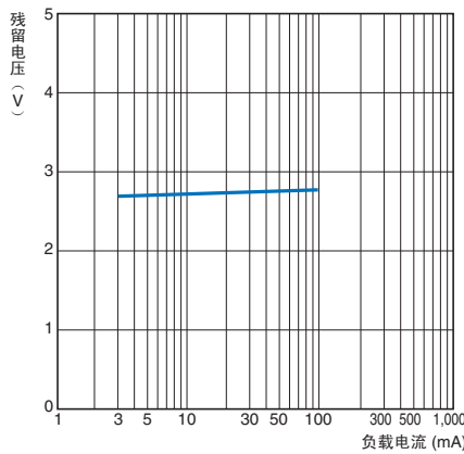
E2EQ-X□D□ (-M1 (T) GJ)
