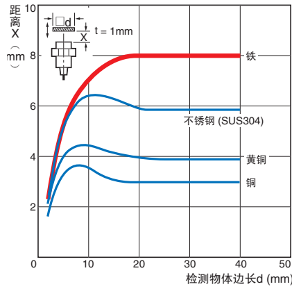
E2EQ-X7D1 (-M1 (T) GJ)
